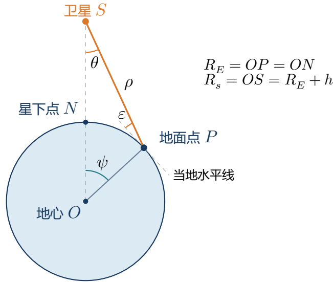
Figure 1: 球形地球上的星地几何：地面仰角、卫星离轴角和地心角。图形不按 GEO 高度比例绘制。
